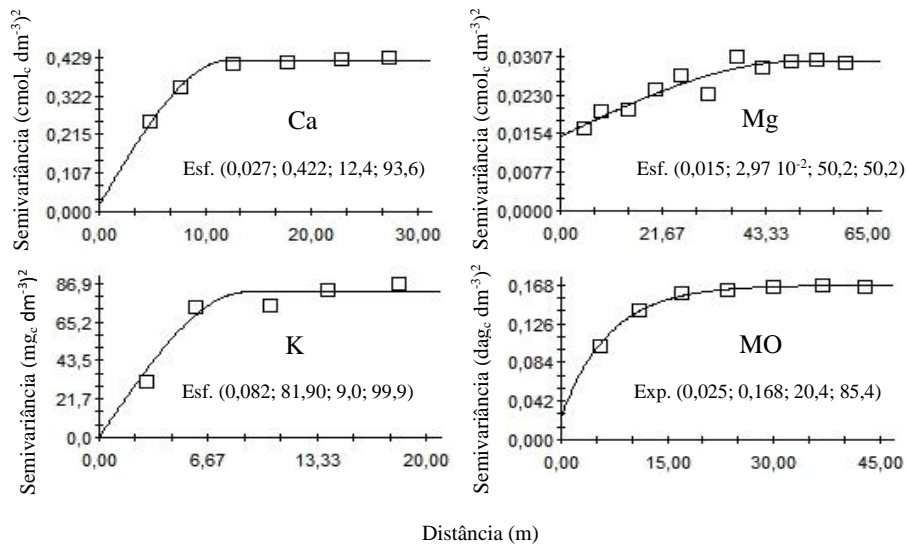
Figura 1 – Modelos de semivariogramas ajustados para cálcio, magnésio, potássio e matéria orgânica em área cultivada com pastagem. Valores entre parênteses são efeito pepita ( C_0 ), patamar ( C_0+C ), alcance (A) em metros e índice de dependência espacial (IDE%), respectivamente. Esf. – modelo esférico; Exp. – modelo exponencial.
