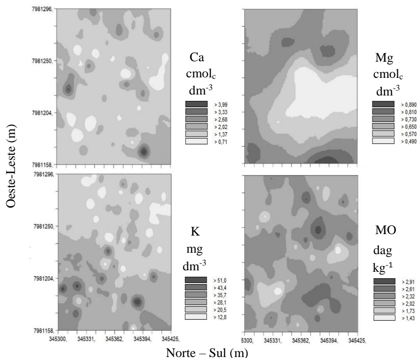
Figura 02 – Mapas de isolinhas das variáveis: cálcio, magnésio, potássio e matéria orgânica em área cultivada com pastagem.
